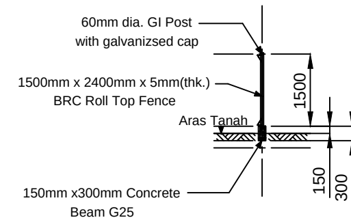
KERATAN A-A
